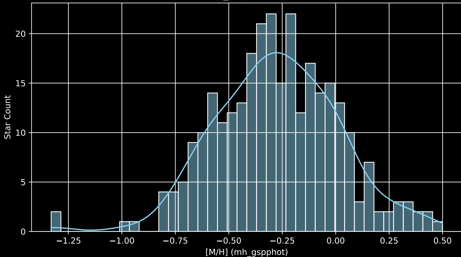
GALAH DR4 Field: [307] [M/H] (mh_gspphot) (n= 290)
