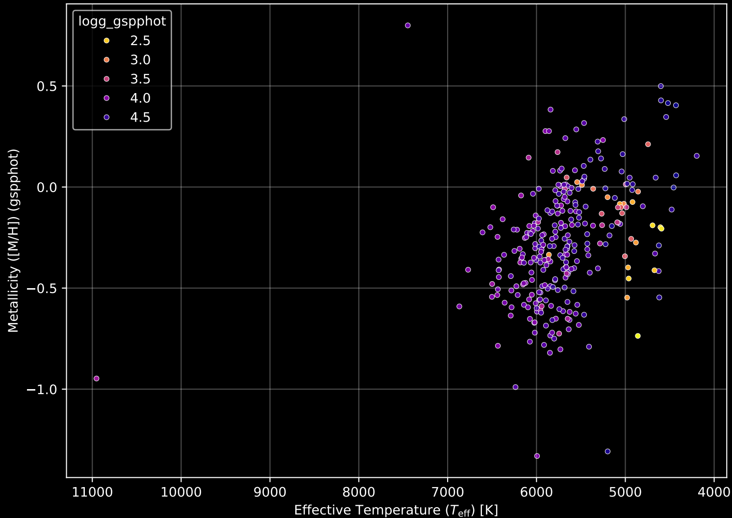
GALAH DR4 Field: [307] Stellar Population Parameters (n= 291)
