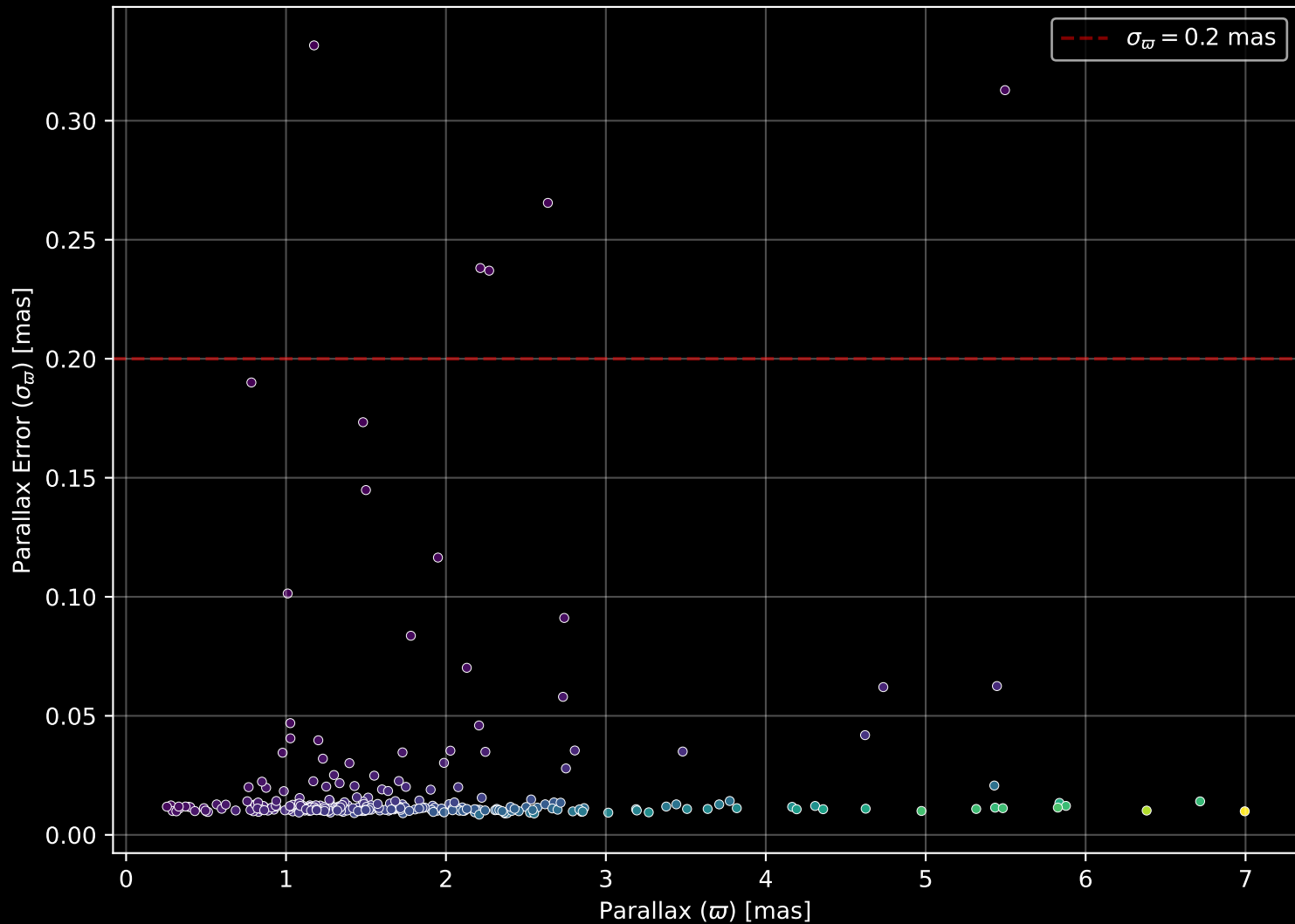
GALAH DR4 Field: [307] Parallax Quality (n= 291)
