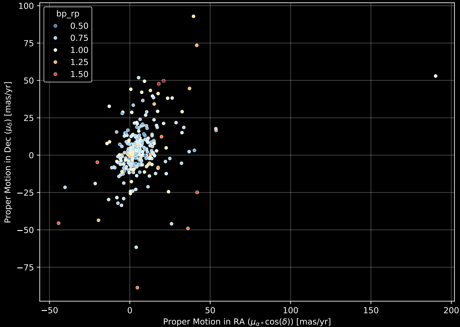
GALAH DR4 Field: [307] Proper Motion Diagram (n= 291)
